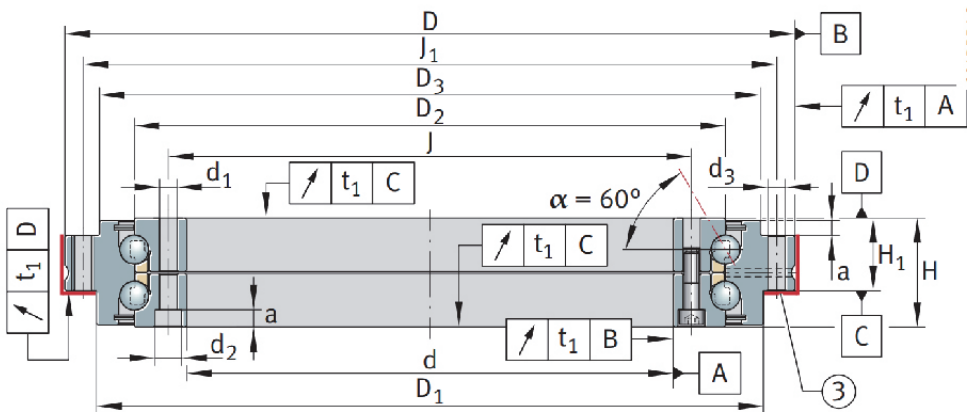
ZKLDF系列、主要尺寸、性能数据
