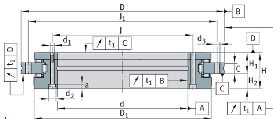
绝对值信号YRTMA轴承尺寸表
